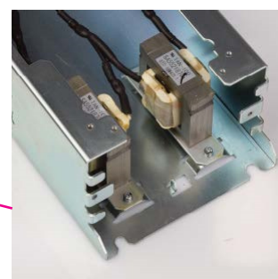
self DC limitant les harmoniques - rendement 98% - filtre CEM intégré déconnectable
